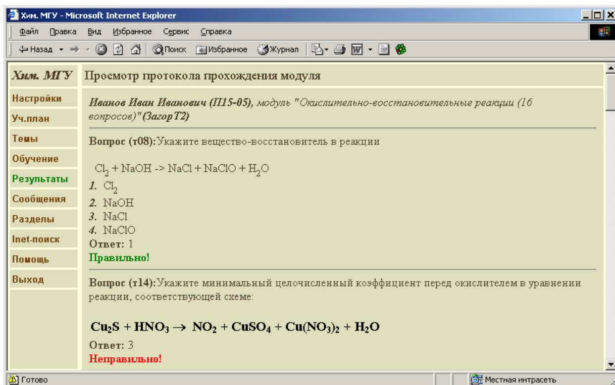
Рис. 13. Протокол тестирования
