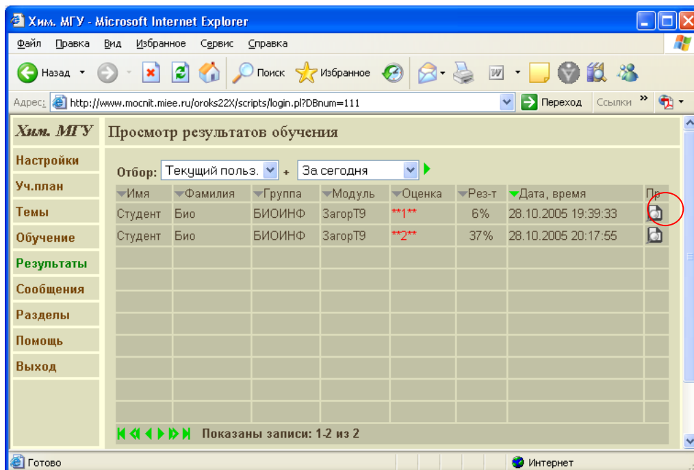
Рис. 12. Результаты обучения
